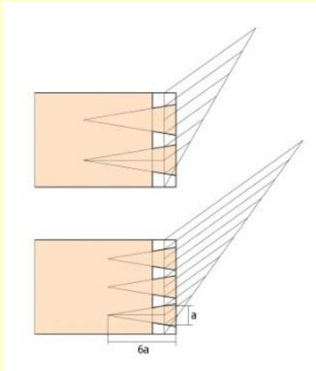
7. ábra: Fecskefarkú fogazás előrajzolása, gyakorlás különböző fogszámmal
