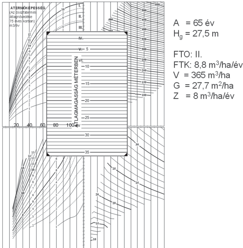
Az ezüst hárs nomogramja (Peszlen 2012)
