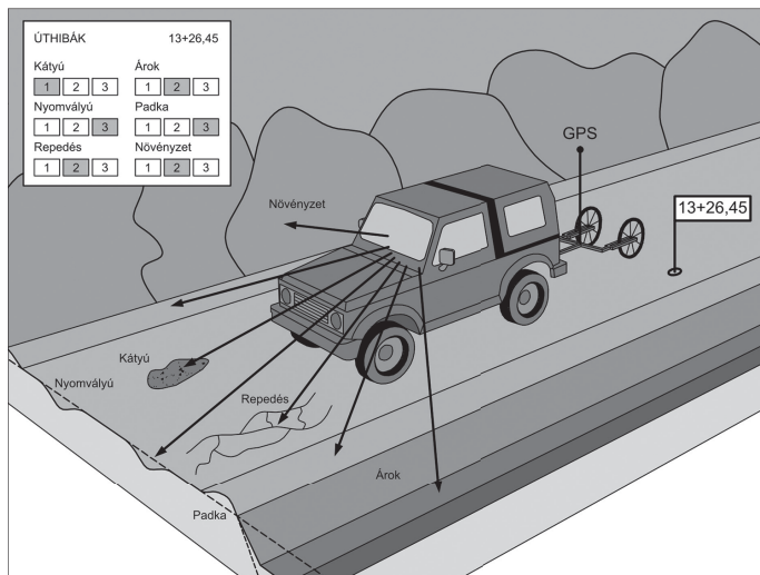
Erdészeti utak szubjektív állapotfelvételére kifejlesztett rendszer
