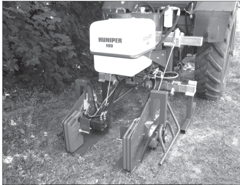
Injektálógép vizsgálata (2009) (Forrás: Soproni Egyetem fotóarchívuma)
