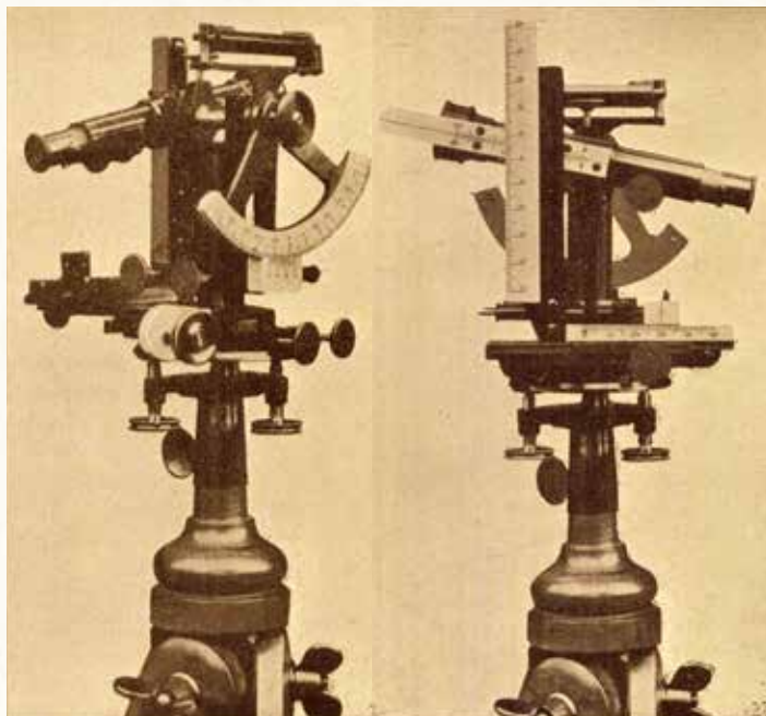
A Fekete–Cséti-féle távcsöves dendrométer (Erdészeti Kísérletek 1905. 7. évf.)
