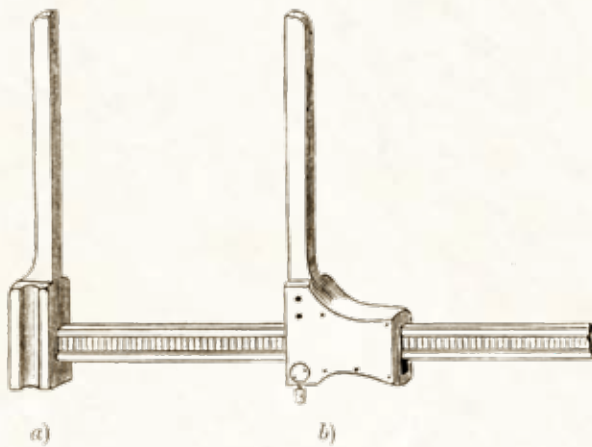
1. ábra. (1/10 term. nagyság.)
