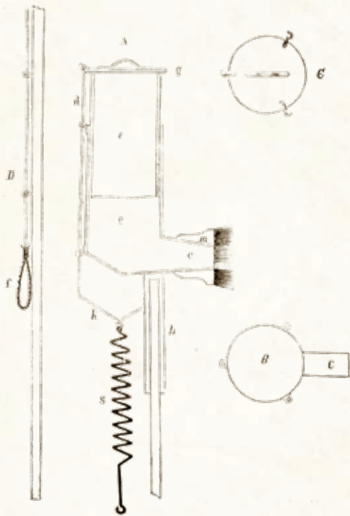
A rúdra erősített, ecset-enyvtartóval ellátott eszköz (Erdészeti Lapok 1891. 30. évf. 11. füzet)
