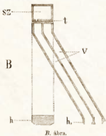
A Fekete-féle tolokás magvető (Erdészeti Lapok 1888. 31. évf. 10. füzet)
